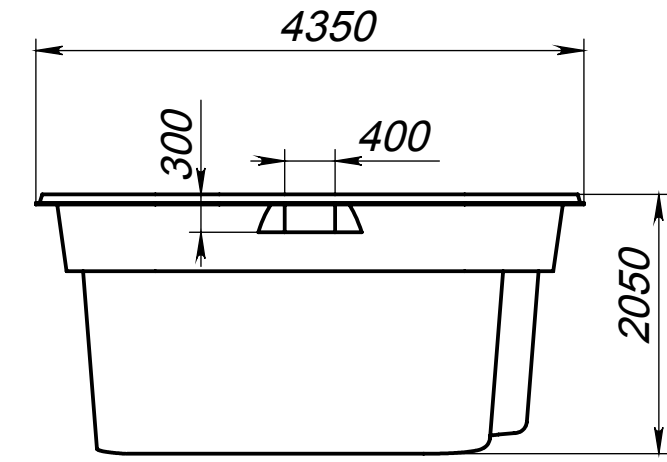
Вид 3-3
