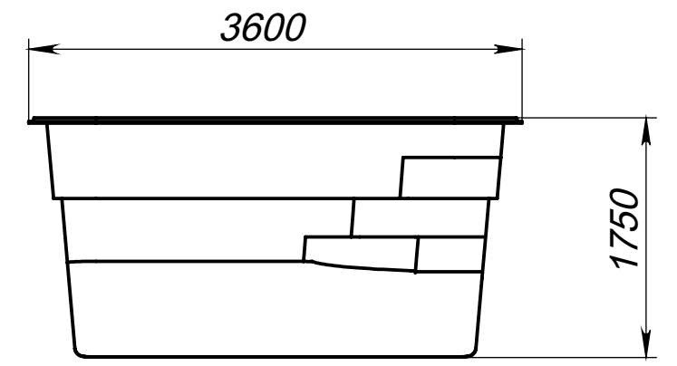
Вид 4-4
