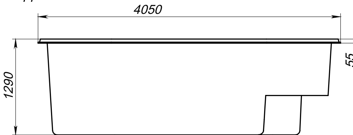
Вид 2-2
