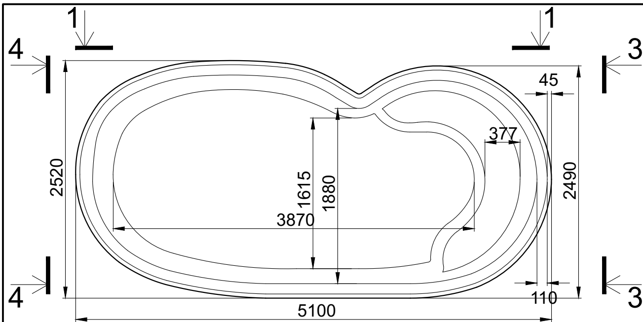
Вид 1-1 5100
