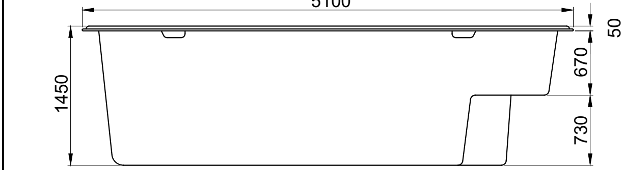
Вид 2-2 5100
